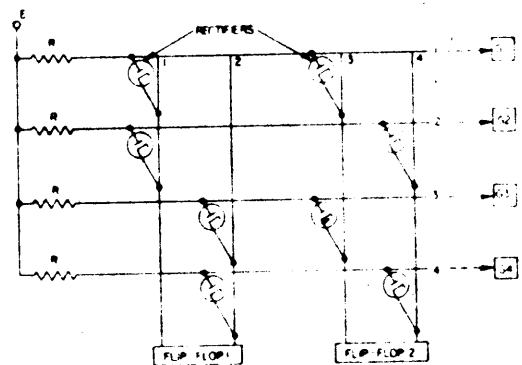
Fig. 13 -Rectifier matrix.
